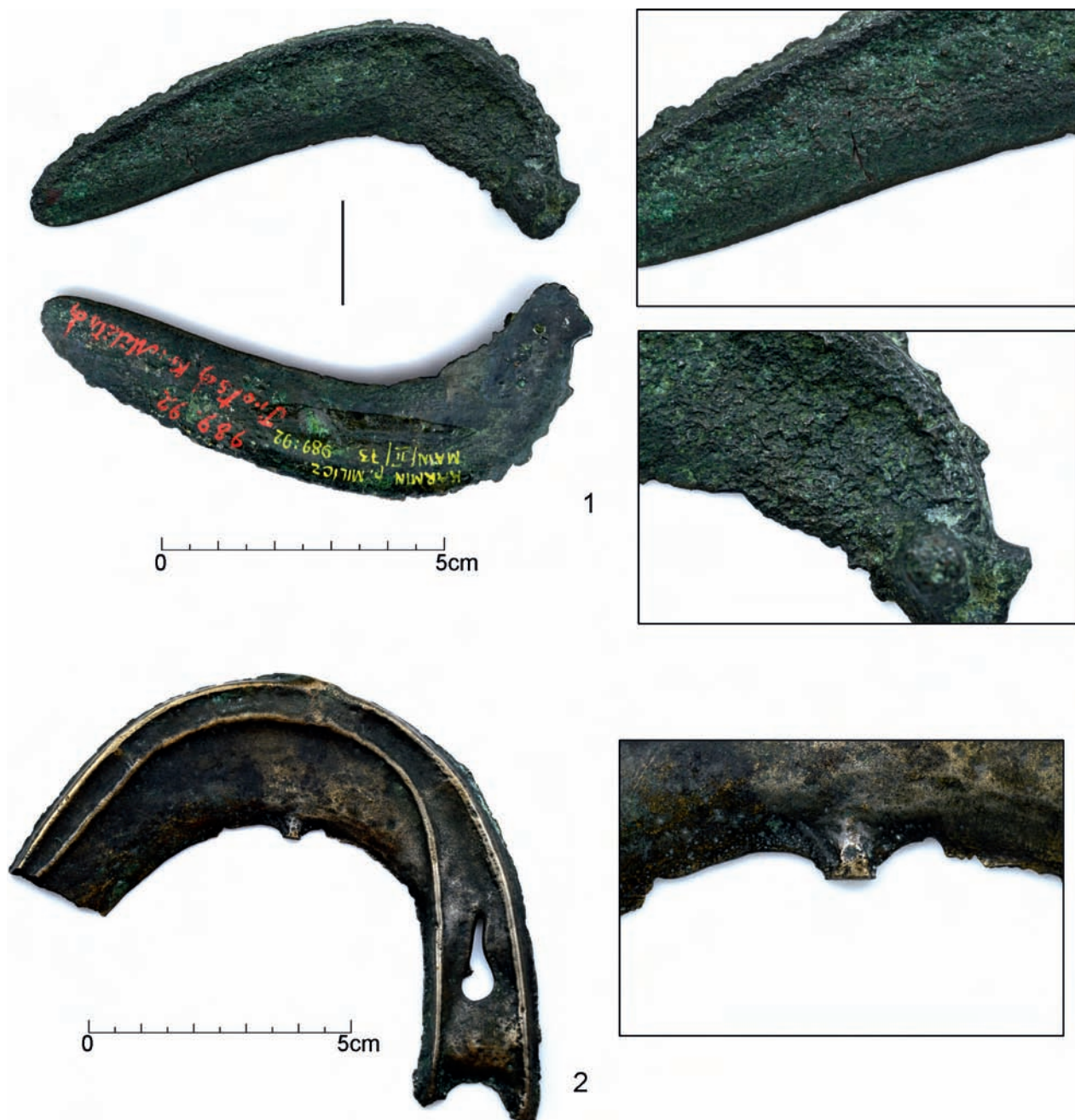
Ryc. 24. Ślady produkcji na przedmiotach metalowych: 1 – sierp nr 73 o powierzchni nierównej (ślad zastygania); 2 – sierp nr 81 z nadlewem/kanałem wlewowym w dolnej partii ostrza.
