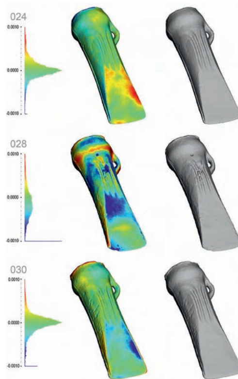
Ryc. 42. Siekierki ze skarbu z Karmina. Porównanie geometrii zabytków 24 i 30, oraz 28 w porównaniu do 24, od lewej: histogram rozkładu wartości, barwne przedstawienie odchyłań na modelu oraz model bez tekstury
