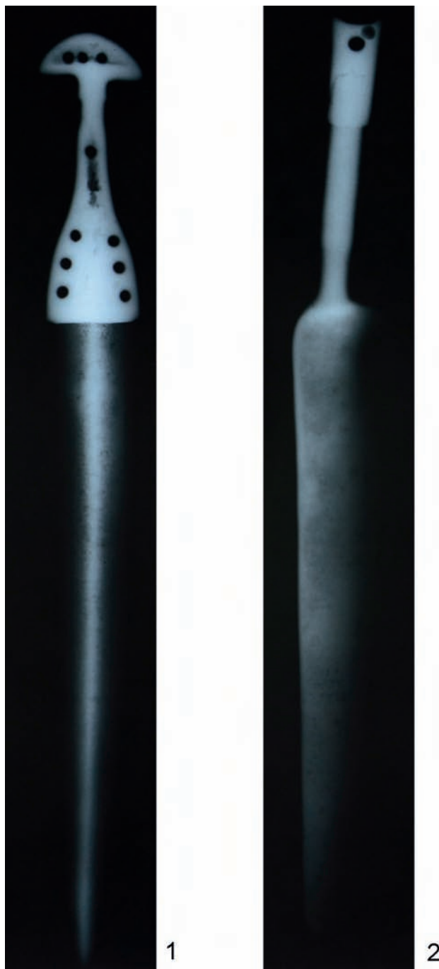
Ryc. 30. Fotografie RTG: 1 – zdjęcie sztyletu nr 40; 2 – zdjęcie noża nr 39. Opr. K. Nowak
