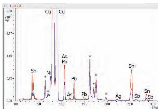
Ryc. 53. Karmin, skarb IV. Widma energetyczne XRF szpil
