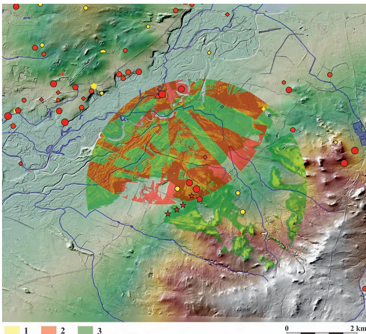
Ryc. 84. Potencjalna widoczność z domniemanej osady – Postolin stan. 2 (analiza wykonana w programie QGIS w wersji 2.18.4 z użyciem wtyczki Visibility analysis for QGIS ver. 0.5.4 – Čučković 2016; maksymalny zasięg widzenia – 2,5 km; wysokość obserwatora – 1,6 m; wysokość obserwowanego punktu – 1 – poziom gruntu, 2 – 0,5 m, 3 – 2 m; legenda ryc. 67; na podstawie tabeli 11; numeryczny model terenu – opracowanie P. Wroniecki; hydrologia na podstawie Komputerowej Mapy Podziału Hydrograficznego Polski udostępnionej w serwisie www.dane.gov.pl z uzupełnieniami. Oprac. graficzne M. Maciejewski
